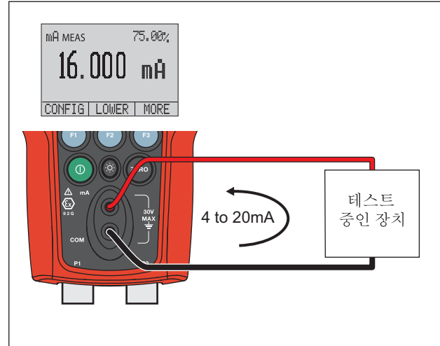
그림 6. 전류 측정
