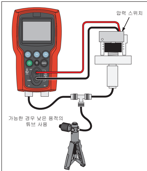
그림3. 압력 스위치 연결
