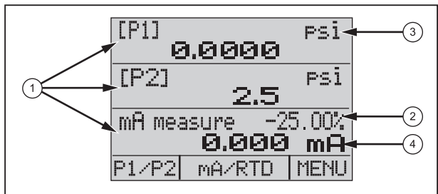
그림 2. 디스플레이
