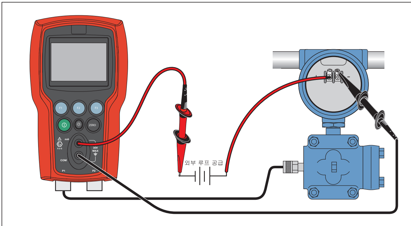
그림 4. 퍼센트 오차 기능 연결
