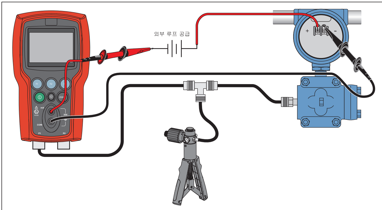
그림 7. 압력-전류 트랜스미터 연결
