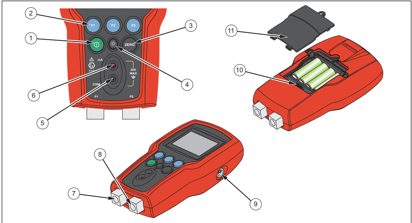
그림1. 제품 인터페이스
